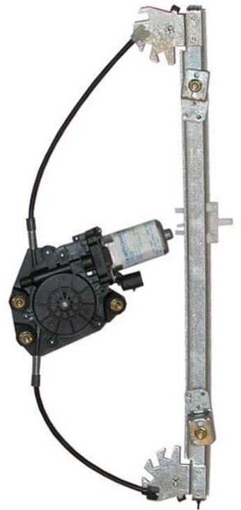
POWER WINDOW LEFT ALZACRISTALLI ELETTRICO SX
